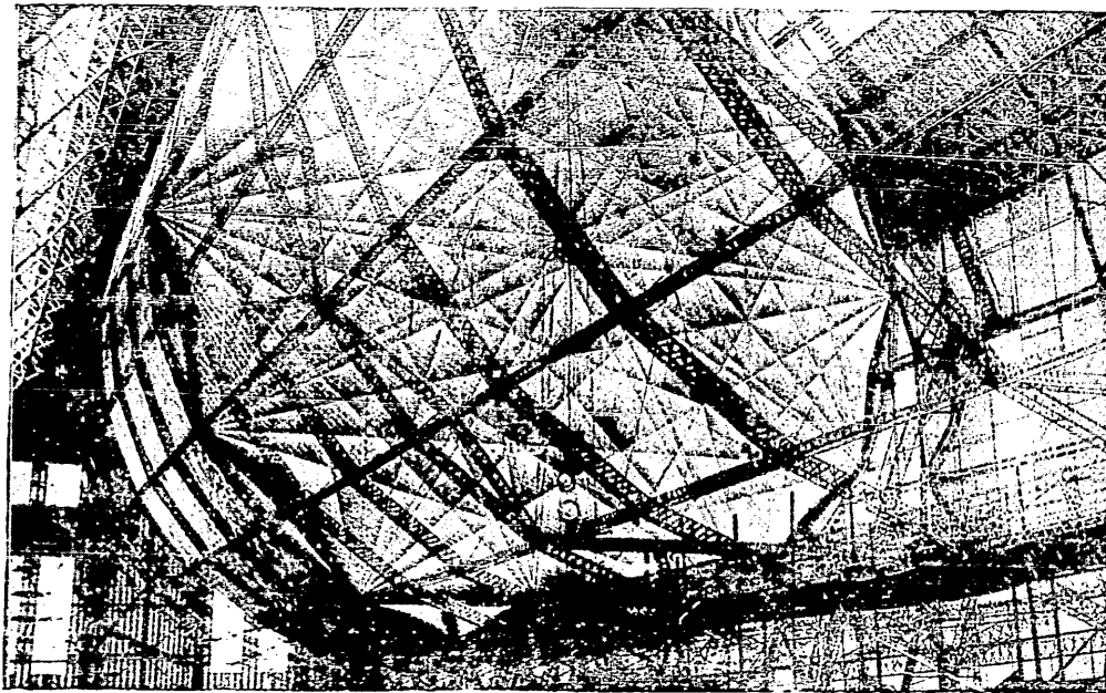
Budowa Zeppelina „Z. R. III.“, który przeleciał z Niemiec do Ameryki.
