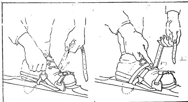
Po przewleczeniu przez kółko, przewija się taśmę spodem podeszwy na drugą stronę buta, okręca go po wierzchu buta i pod podeszwą wraca do sprzączki, na którą zapina się ostecznie.
