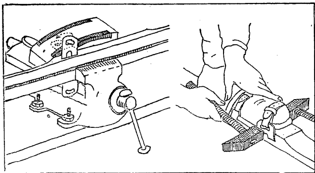
1) Nartę wraz z formą umieszczoną w odpowiednim punkcie narty, chwytając się w silny warsztat i zginając szcękę z pomocą drewnianego młota. 2) Ostateczne poprawki zgięcia za pomocą młotków.
