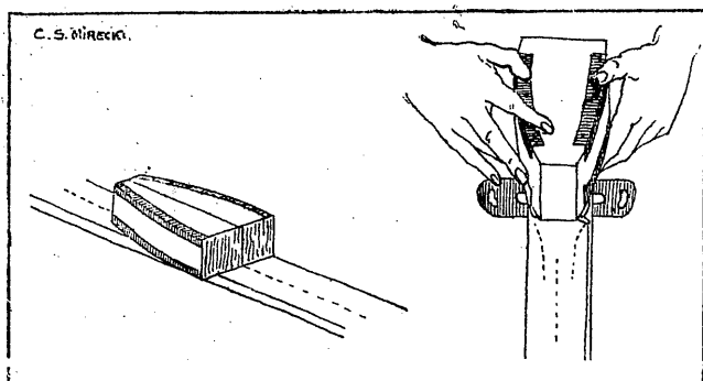
Formy służące do gięcia szcęk przy nartach. Rozcięcie formy wzdłuż pozwala przez użycie wkładek, do użycia dla rozmaitych wielkości obuwia narciarskiego.
